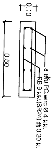
รูปตัดขวาง
